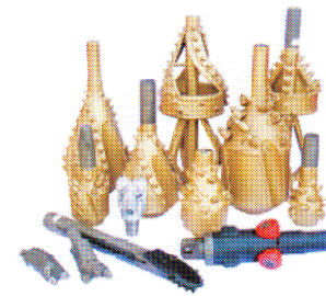
Bohrzubehör für HDD-Bohranlagen
